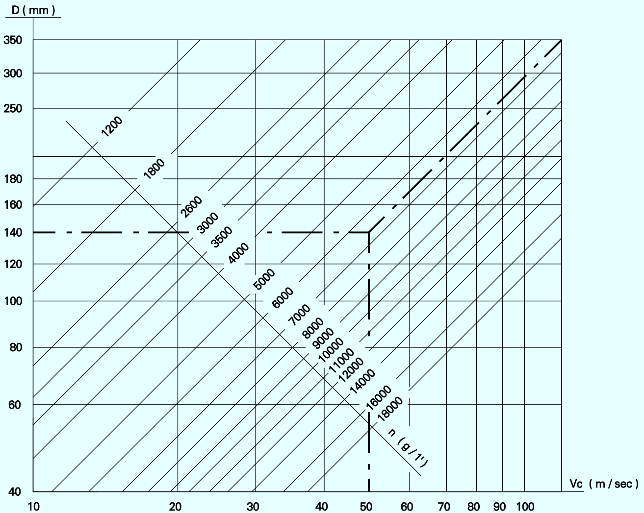
DIAGRAMMA PER RILEVARE IL NUMERO DEI GIRI DEGLI UTENSILI IN RAPPORTO AL DIAMETRO ED ALLA VELOCITA' DI TAGLIO PRESCELTA.
